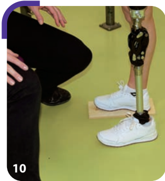
Controle van de juiste hoogte van de prothese
